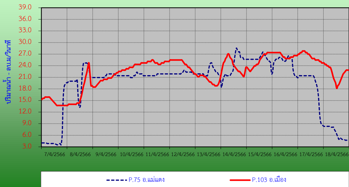
กราฟแสดงปริมาณน้ำปิ้งรายชั่วโมงรอบวันที่ 14-15/2566 ที่สถานีแม่น้ำปิง (P.75) บ้านข่อแล อ.แม่แตง และที่สถานีแม่น้ำปิง (P.103) บ้านป่าข่อยใต้ อ.เมือง จ.เชียงใหม่
